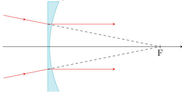
Lentille divergente
