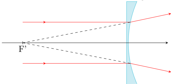
Lentille divergente
